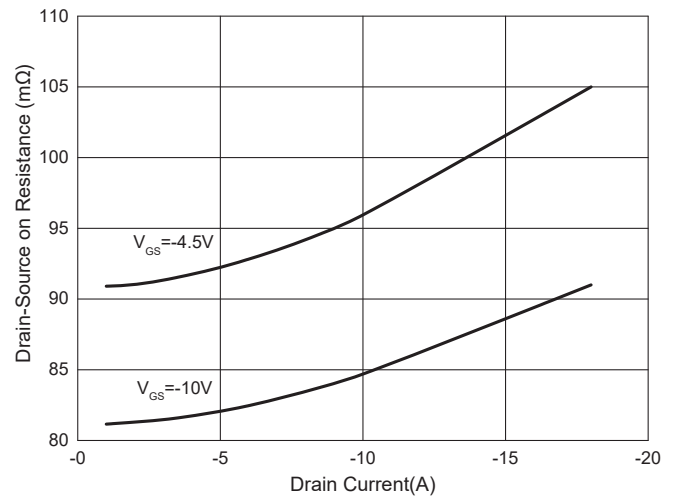
Fig. 8 - R_{DS(ON)} - I_D
